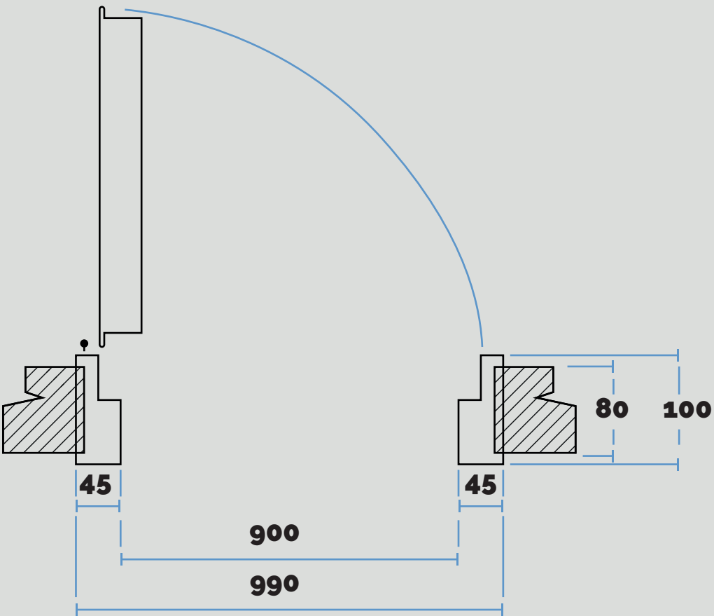
Corte horizontal del marco
