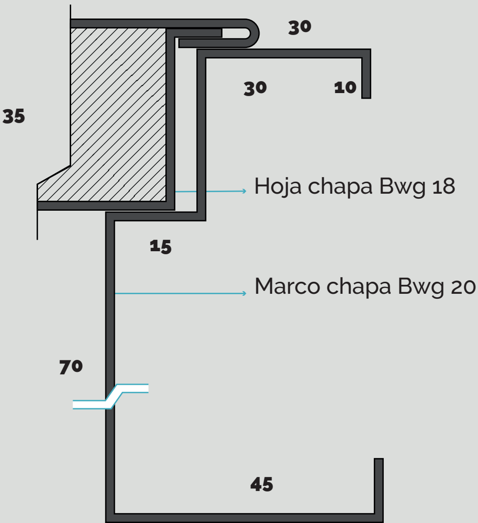
Corte horizontal del marco
