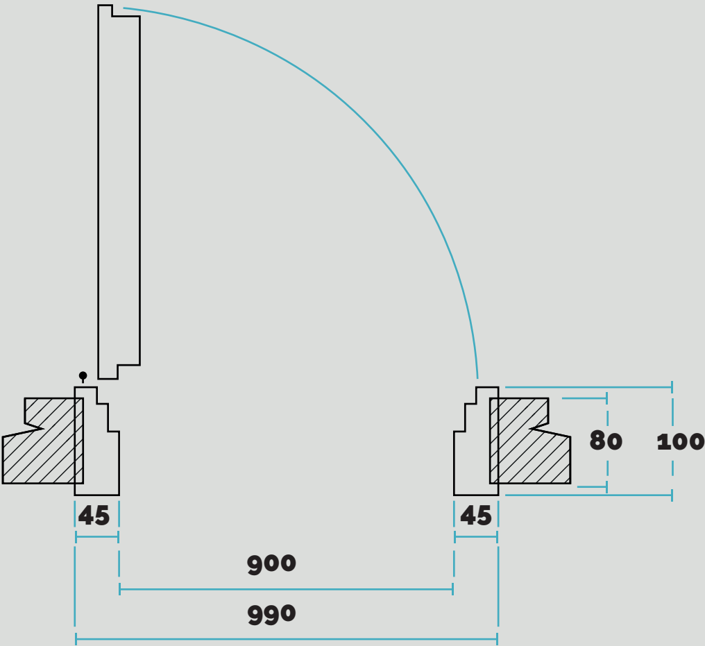
Corte horizontal del marco
