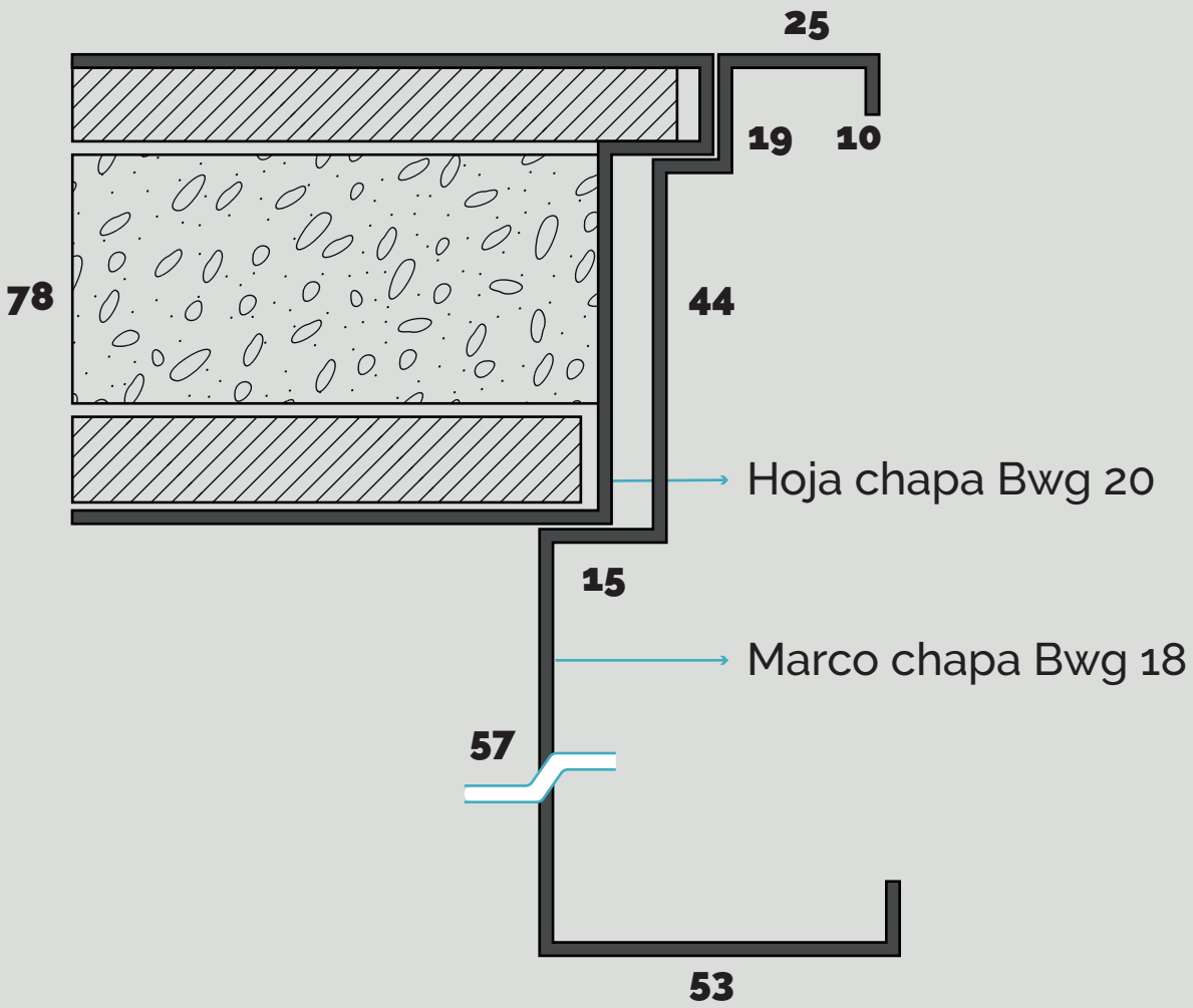
Corte horizontal del marco
